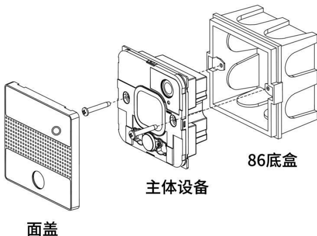
图 3-3（安装演示）
